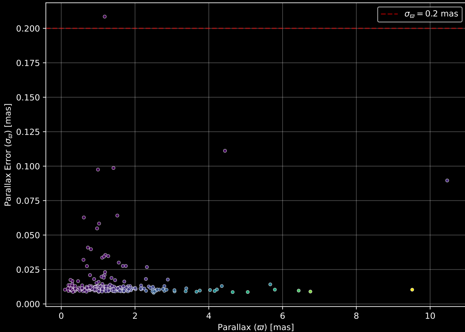
GALAH DR4 Field: [2263] Parallax Quality (n= 261)
