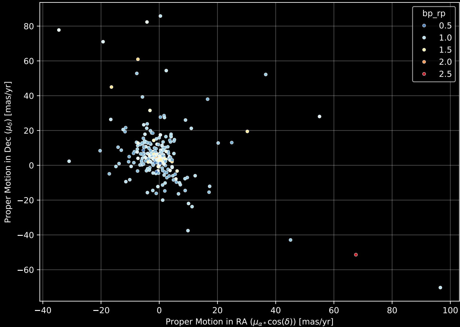
GALAH DR4 Field: [2263] Proper Motion Diagram (n= 261)
