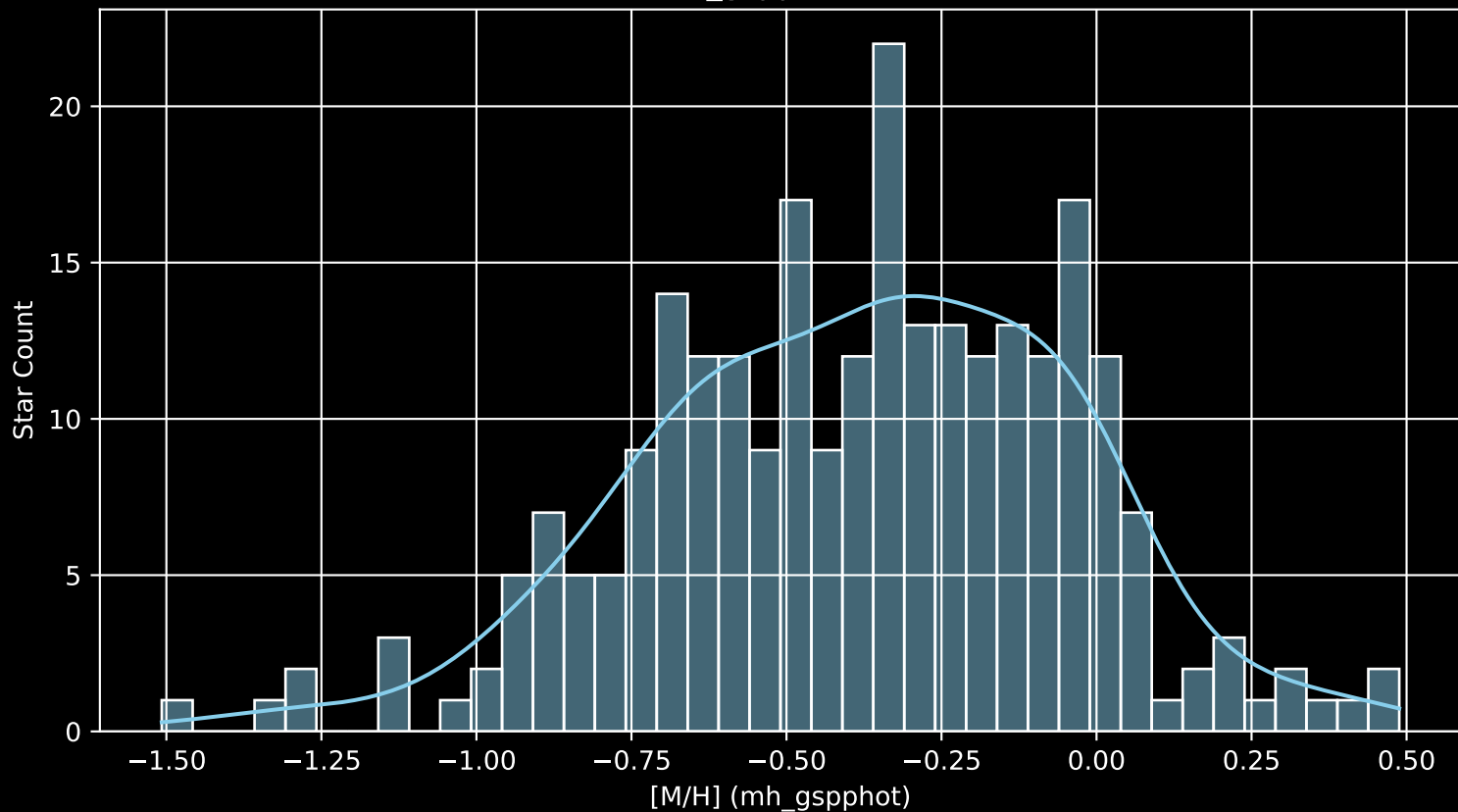
GALAH DR4 Field: [2263] [M/H] (mh_gspphot) (n= 260)
