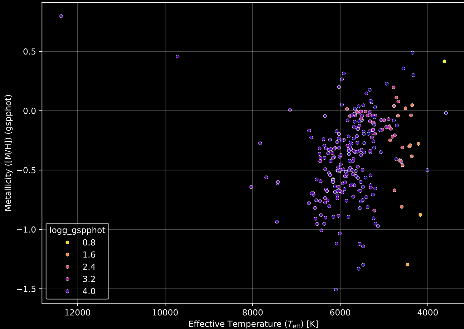
GALAH DR4 Field: [2263] Stellar Population Parameters (n= 261)
